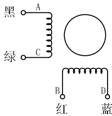
42BYGHM101 42BYGHM403
