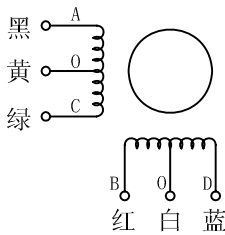
42BYGHM107
