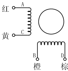
42BYGHM023
