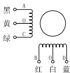
42BYG015 42BYG401 42BYGH102 42BYGH107 42BYGH404
